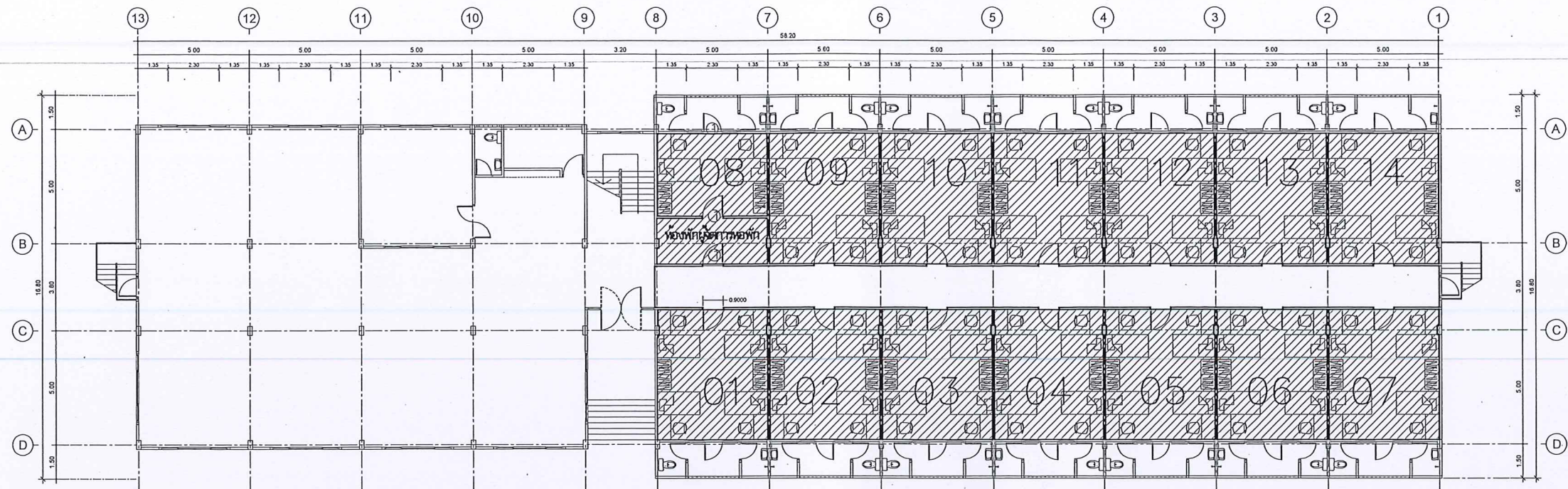
แปลนชั้น 1 อาคารหอพัก 3
