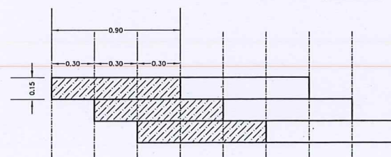
ปูพื้นกระเบื้องยางไม้เทียมกันแบบ 1:3
