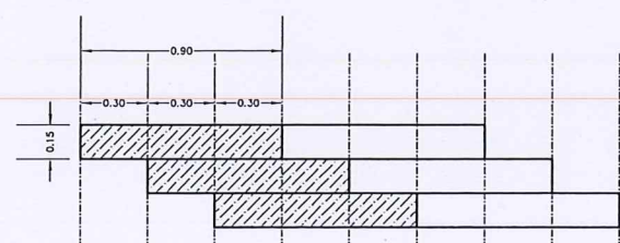
ปูพื้นกระเบื้องยางไม่เหลื่อมกันแบบ 1:3
