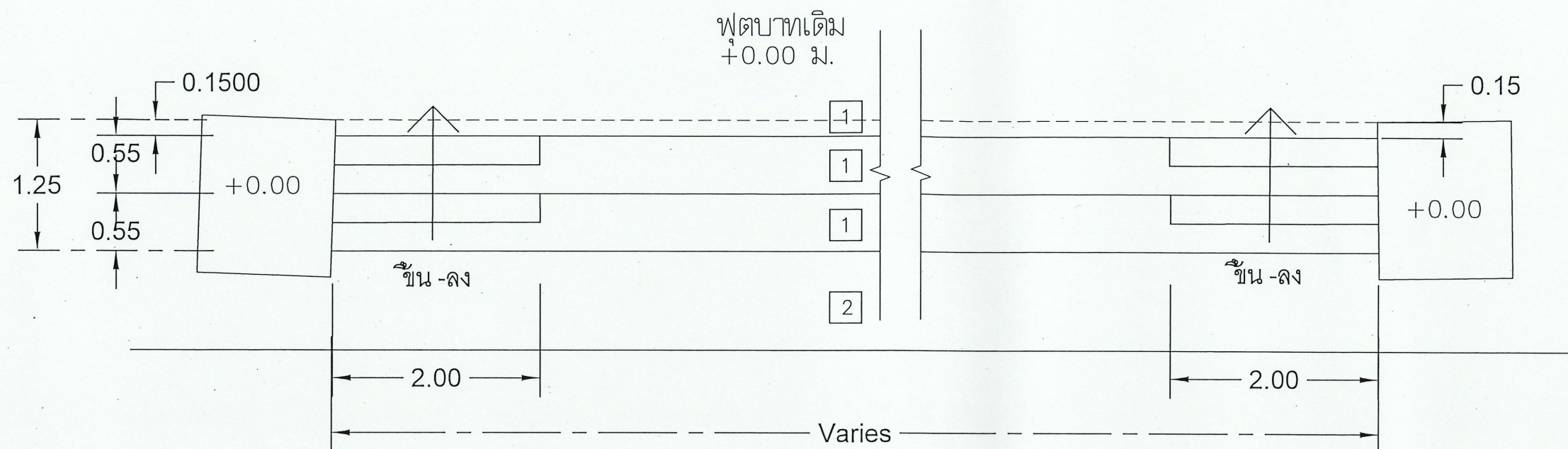
แปลนขยายที่หนึ่ง ค.ส.ล.1 มาตราส่วน 1:50
