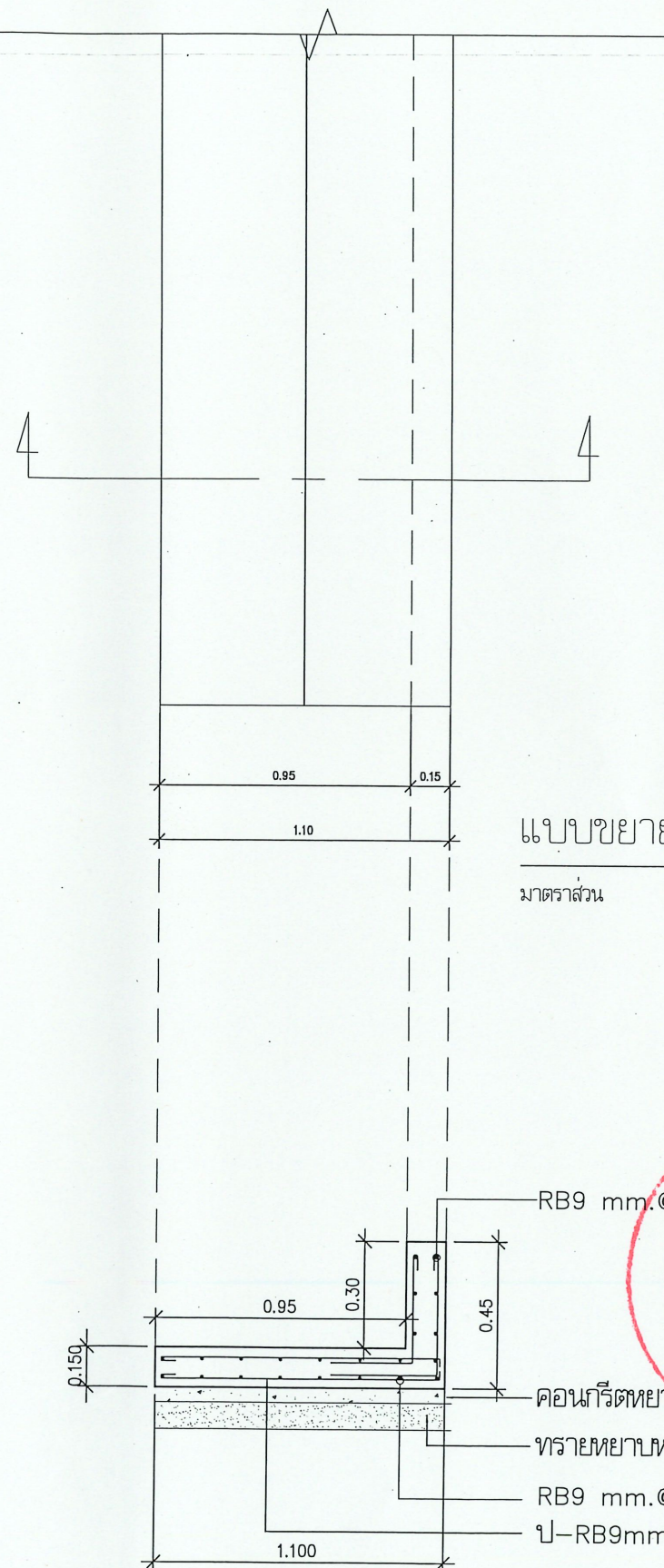
แบบขยายรูปตัดโครงสร้างที่ 2 ค.ส.ล. 2
