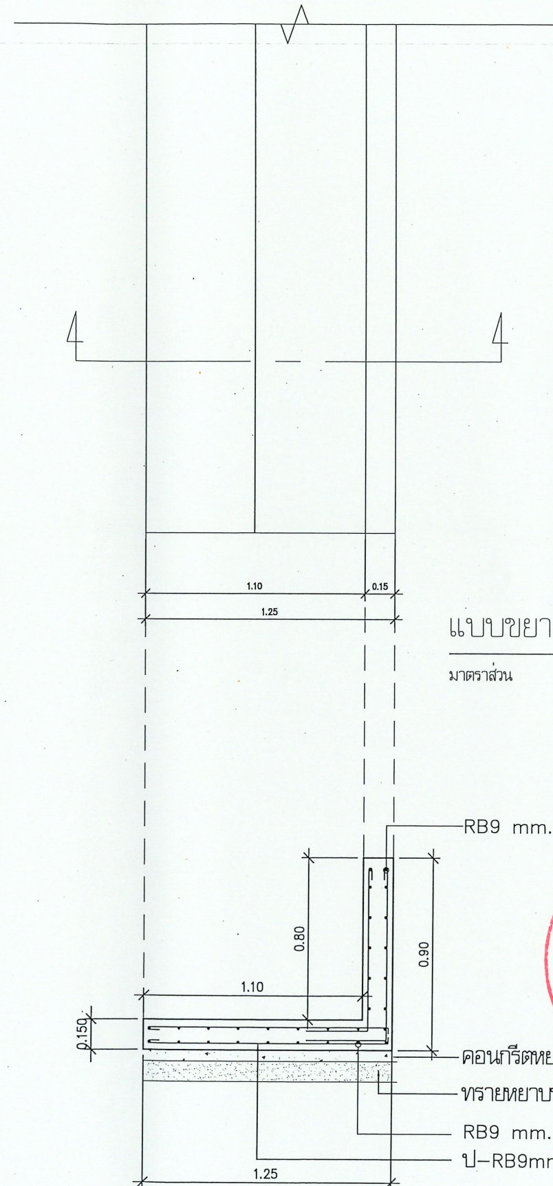
แบบขยายรูปตัดโครงสร้างที่นิ่ง ค.ส.ล. 1
