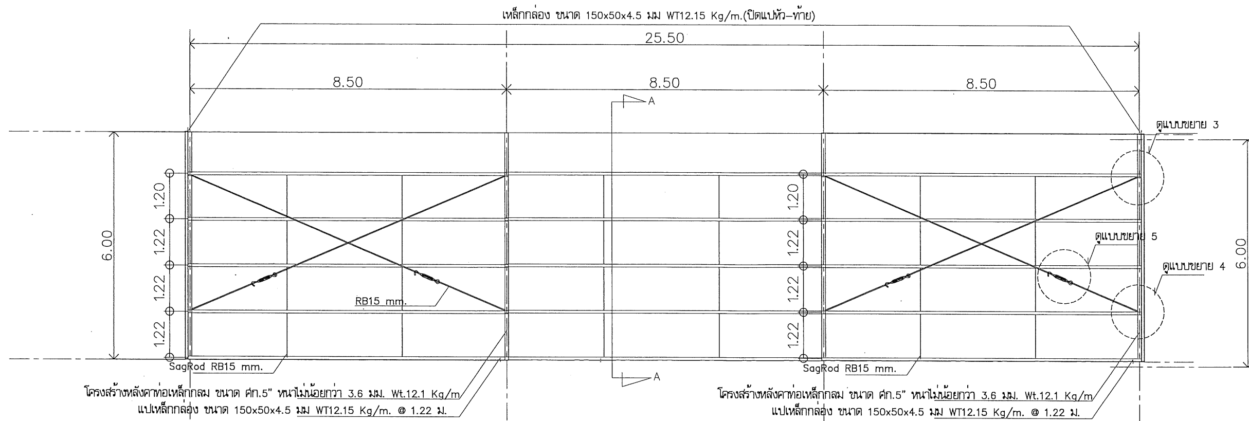
แปลนโครงสร้างหลังคา มาตราส่วน 1:100
