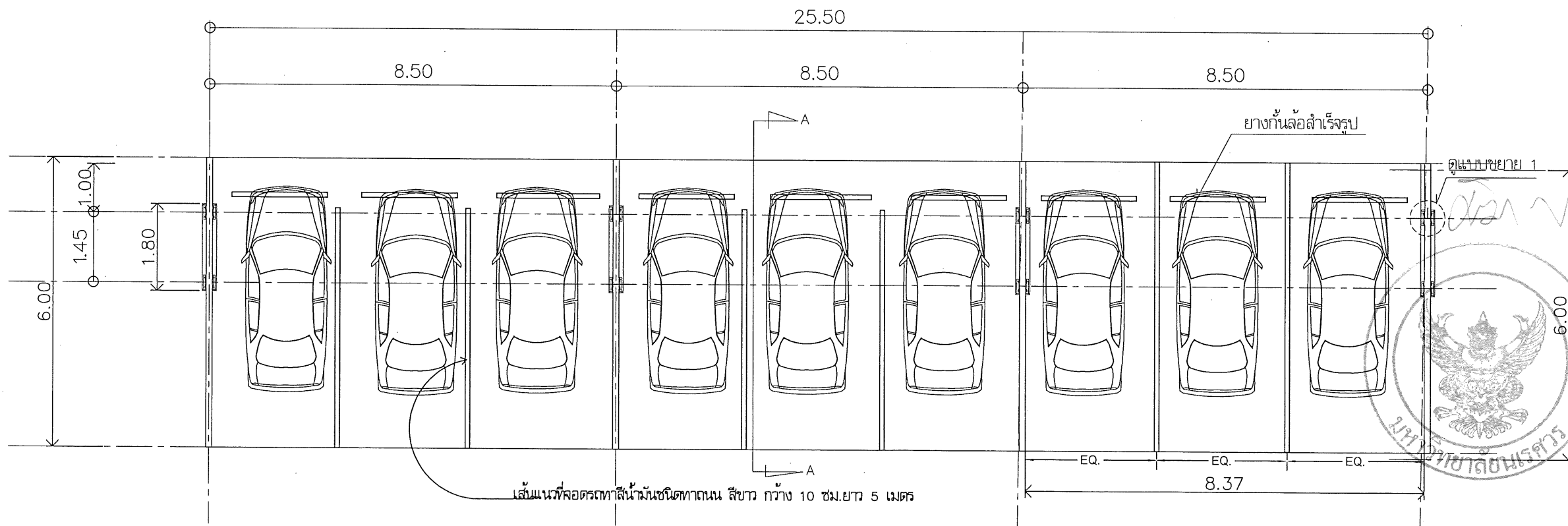
แบบแปลนที่จอดรถยนต์ มาตราส่วน 1:100
