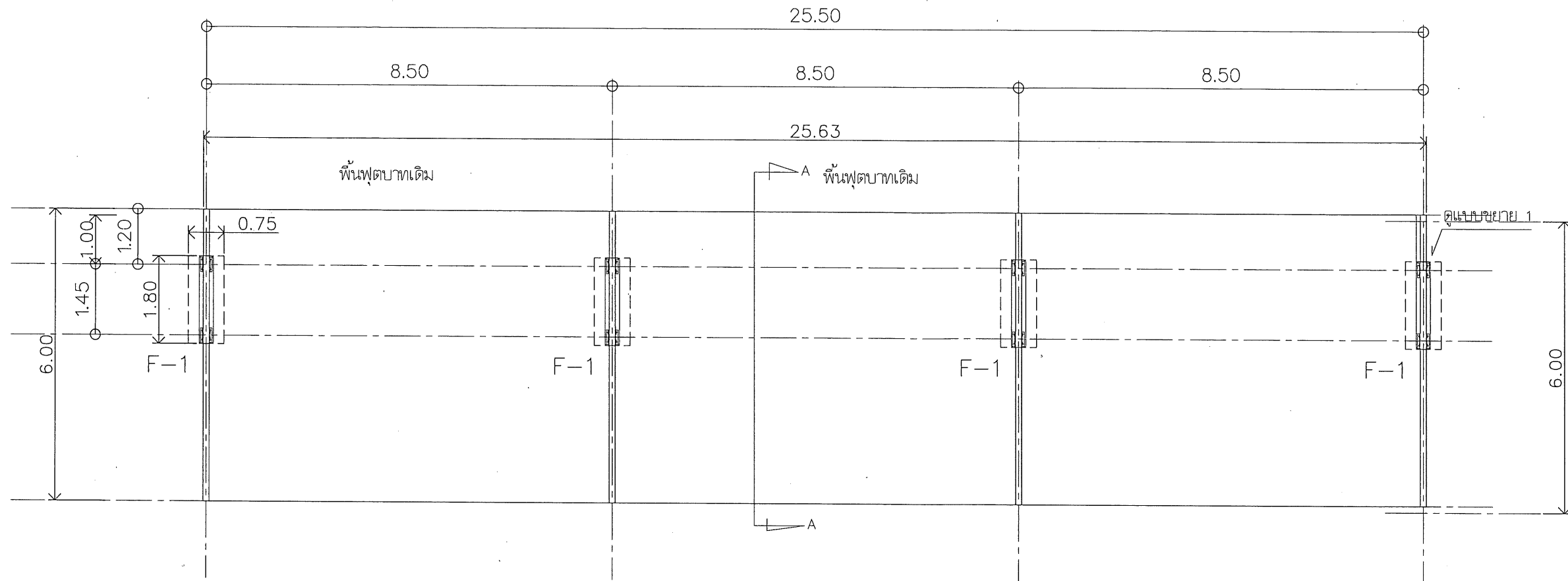
แปลนฐานราก มาตราส่วน 1:100
